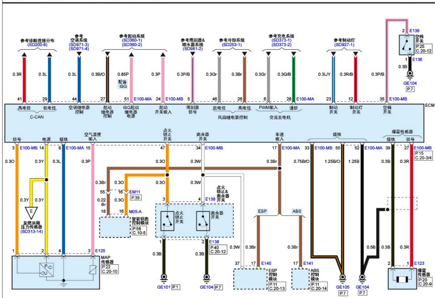
发动机控制系统(G4LC : KAPPA 1.4L MPI M/T)(8)
